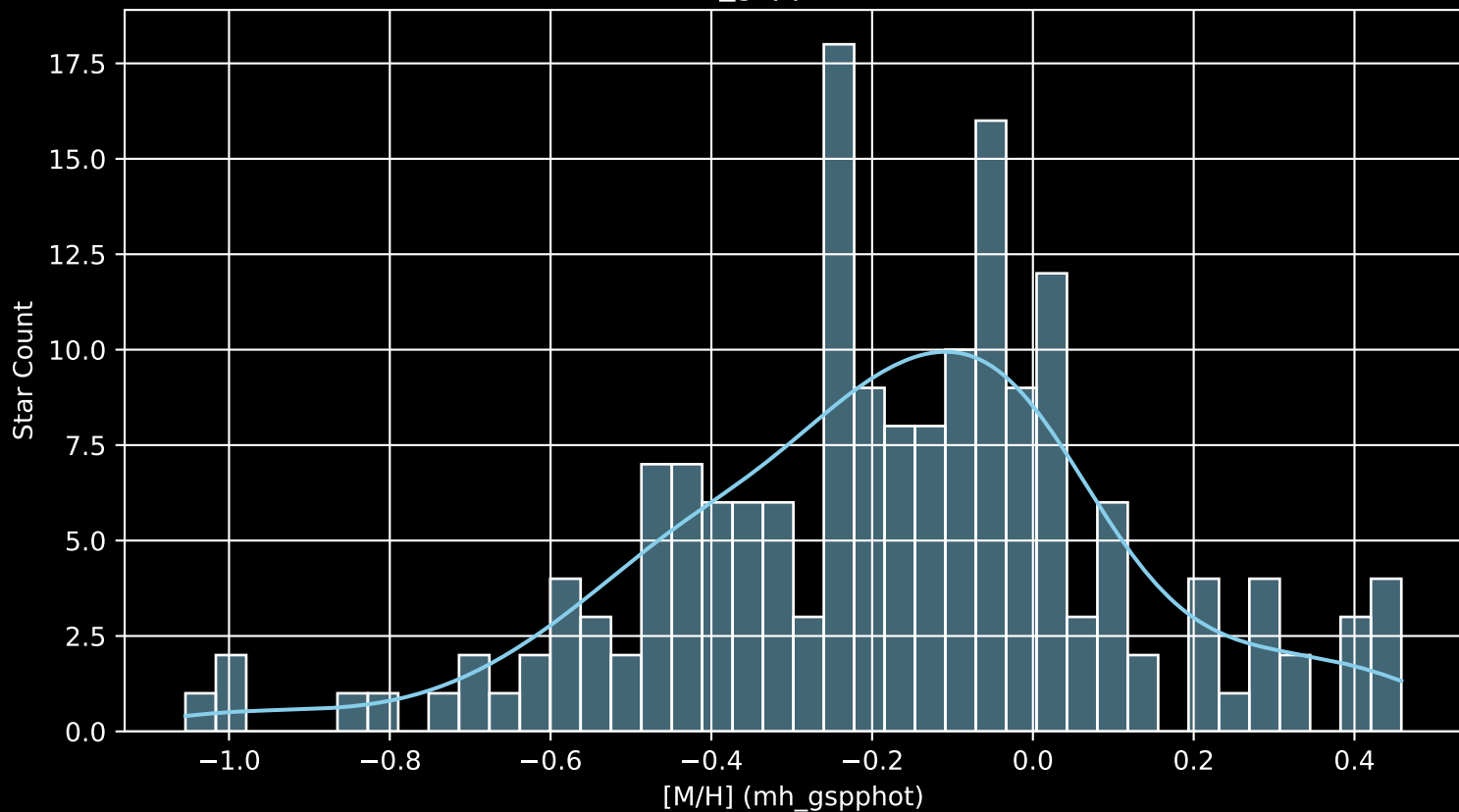
APOGEE DR17 Field: [056+39 MGA [M/H] (mh_gspphot) (n= 174)
